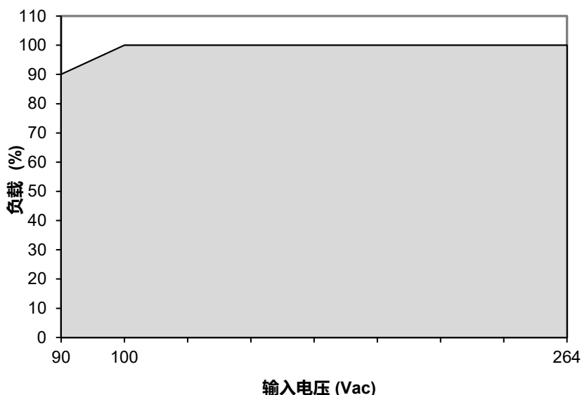
图. 2 AC 输入电压功率降额
